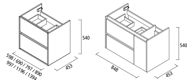
Mueble 2 cajones
